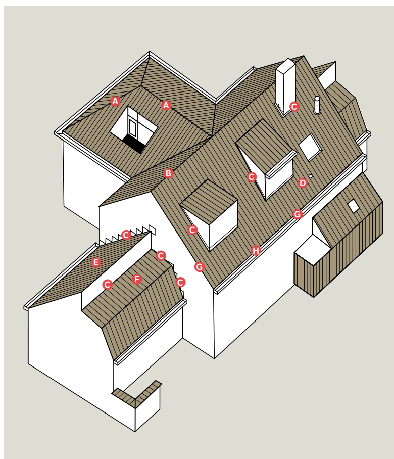
A B sous-faîtières de ventilation
