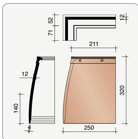
PELF8800 3,6 pièces/m crt Pièce d'angle gauche (bardage)
