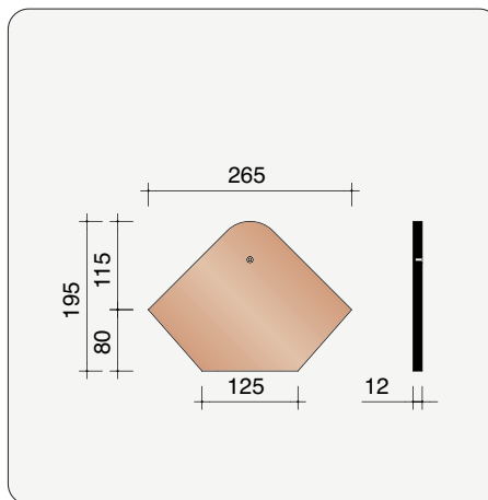
P0002842 Fronton pour faîtière angulaire sans emboîtement 45°
