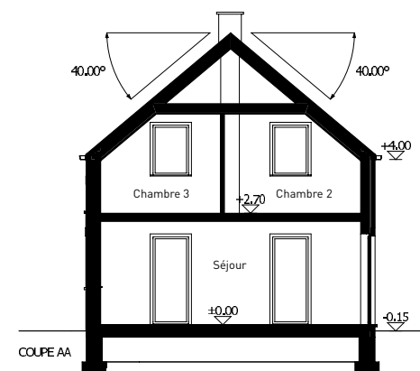
VUE EN COUPE
