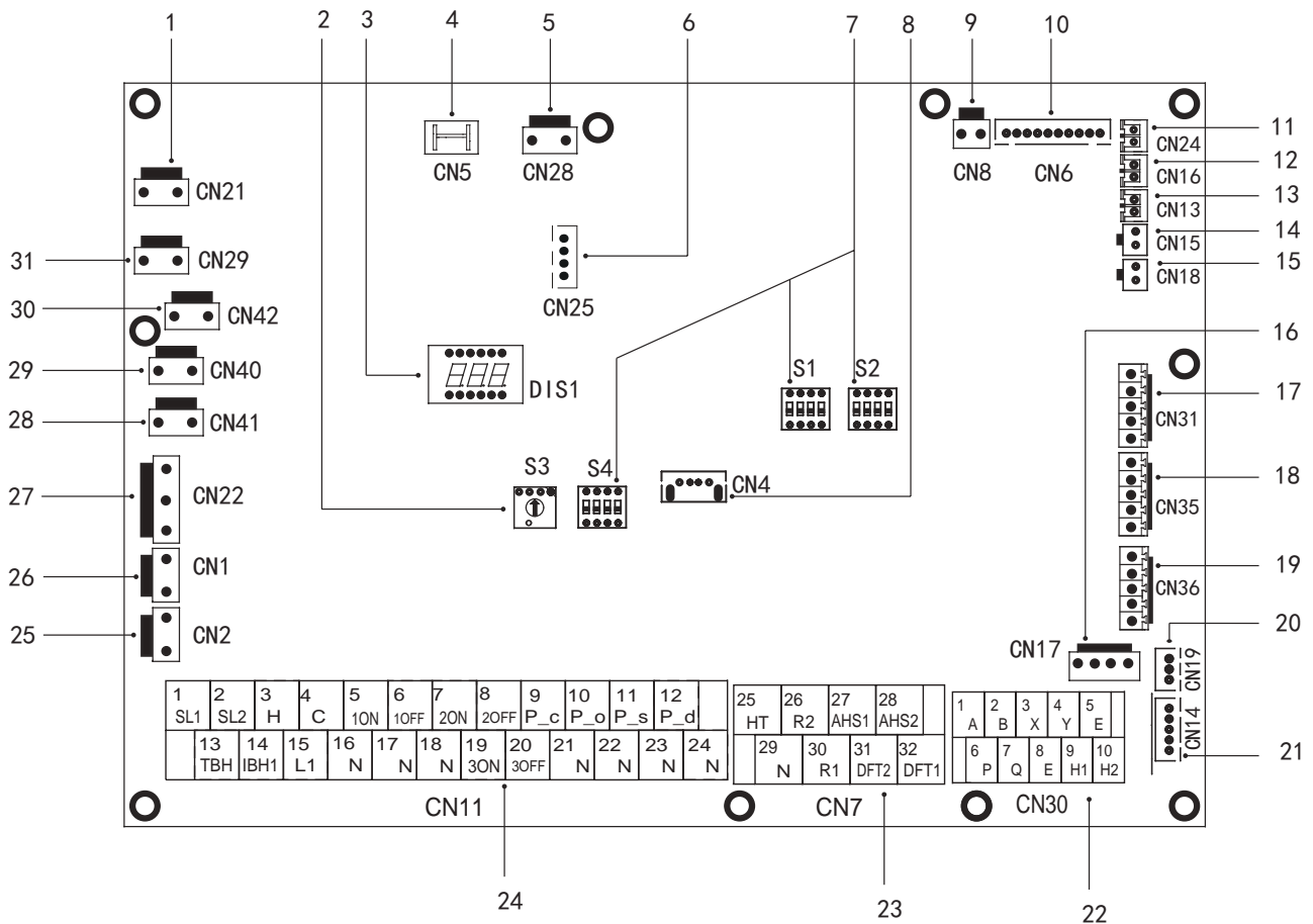
fig. 21 - Carte hydrothermique
