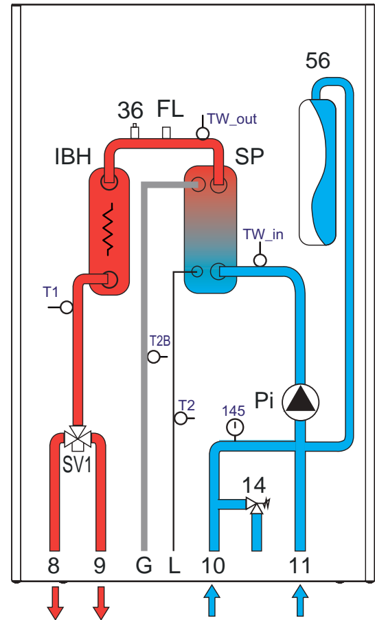
fig. 5 - Schéma hydraulique unité intérieure
