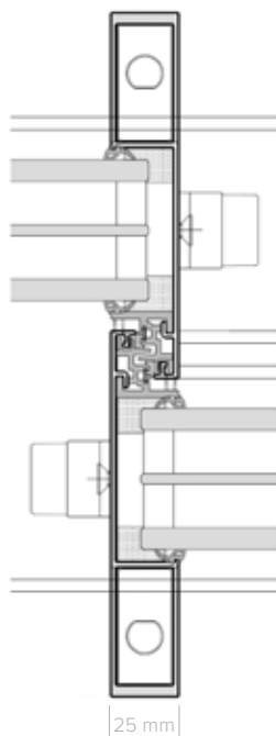
Profilé section centrale
