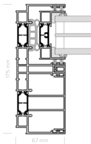
Profilé dans le mur
